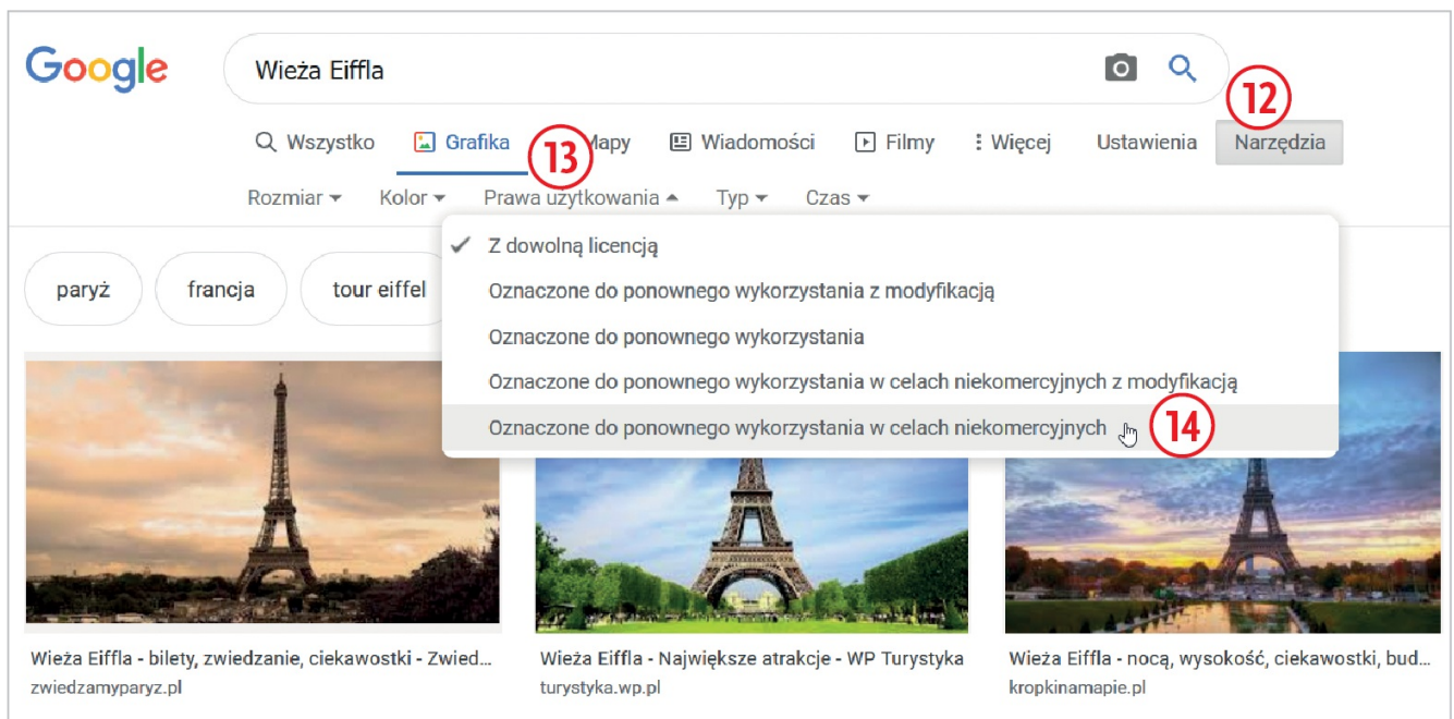
Rys. 6. Wybór licencji
